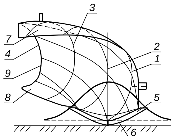
Рис. 3. Схема лемішно-полицевого картоплекопача, вид робочої поверхні
