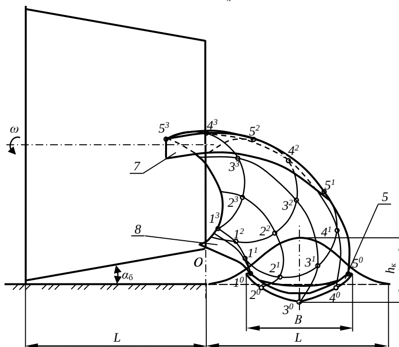
Рис. 6. Схема лемішно-полицевої робочої поверхні
