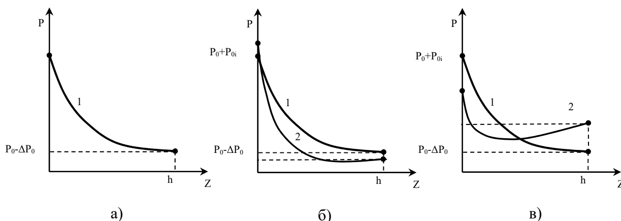
Рисунок 1. Якісна залежність рівноважного розподілу суміші газів в закритому приміщенні: а – барометричний розподіл (повітря); б – суміш повітря і більш важкого газу ( \text{CO}_2 ); в – суміш повітря і легкого газу.
