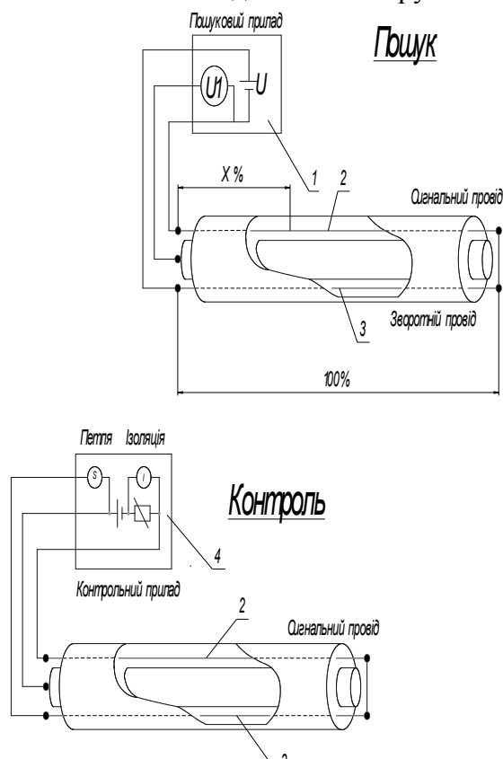
Рис. Локалізація місцезнаходження дефекту: 1- пошуковий прилад; 2 – сигнальний провід; 3 – зворотний провід; 4 – контрольний прилад; X% – результат пошуку у відсотках.
