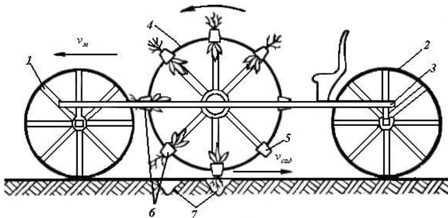
Рисунок 6 – Схема роботи розсадосадильної машини СКН-6А: 1, 2 – ходові колеса; 3 – рама; 4 – садильний диск; 5 – розсадотримач; 6 – саджанці; 7 – борозна для саджанців.
