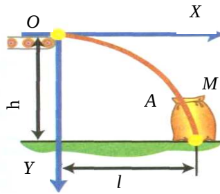
Рисунок 7 – Схема руху зерна у зерновому металнику
