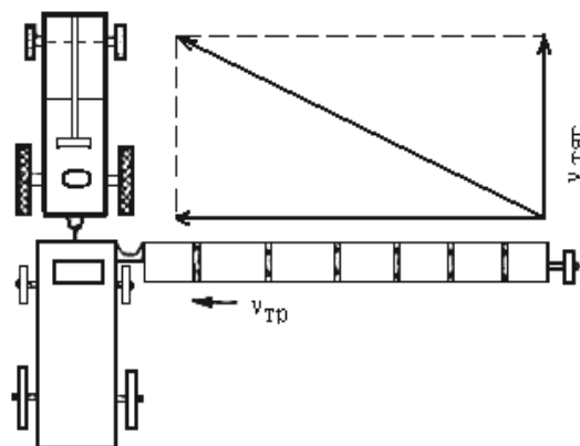
Рисунок 3 – Додавання рухів: v_{тр} – швидкість транспортера; v_{тяг} – швидкість тягача
