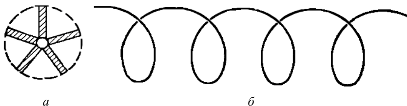
Рисунок 1 – Траєкторія руху точок лопатей мотовила під час руху комбайна: а – у системі відліку, яка пов'язана з корпусом комбайна; б – відносно спостерігача, який стоїть на землі
