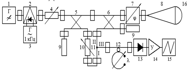
Рис. 1. Блок-схема измерительной установки: 1 – генератор на ЛПД; 2 – p-i-n модулятор; 3 – звуковой генератор с частотой 1 кГц; 4 – аттенюатор установочный; 5, 6 – направленные ответвители; 7 – фазовращатель; 8 – гофрированный конический облучатель; 9 – согласованная нагрузка; 10 – аттенюатор поляризационный; 11 – волноводный тройник; 12 – волномер; 13 – детекторная секция; 14 – усилитель резонансный; 15 – осциллограф; 16 – обтекатель
