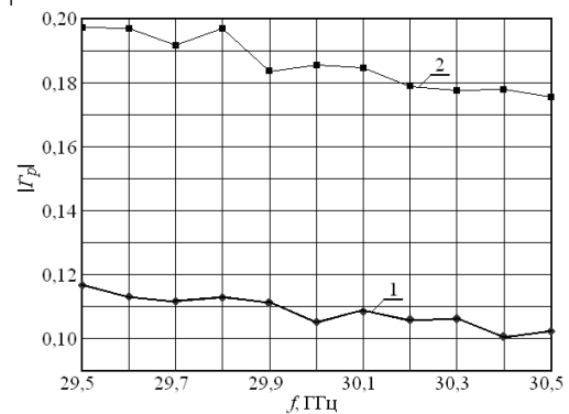
Рис. 2. Экспериментально измеренный |\dot{\Gamma}_p| от раскрыва рассчитанного гофрированного конического облучателя без обтекателя и с ним
