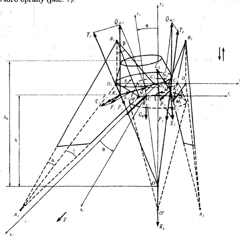
Рис. 1. Силова схема вібраційного викопування коренеплоду з ґрунту
