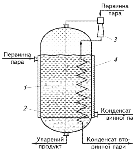
Рис. 2. Схема випарного апарата з циркуляційним контуром рекуперації випару: 1 — випарний апарат; 2 — сорочка випарного апарата; 3 — термоежекторний апарат; 4 — конденсатор вторинної пари
