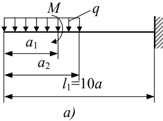
Рисунок 7.1 – Розрахункові схеми
