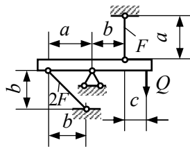
Рисунок 4.1 – Розрахункові схеми
