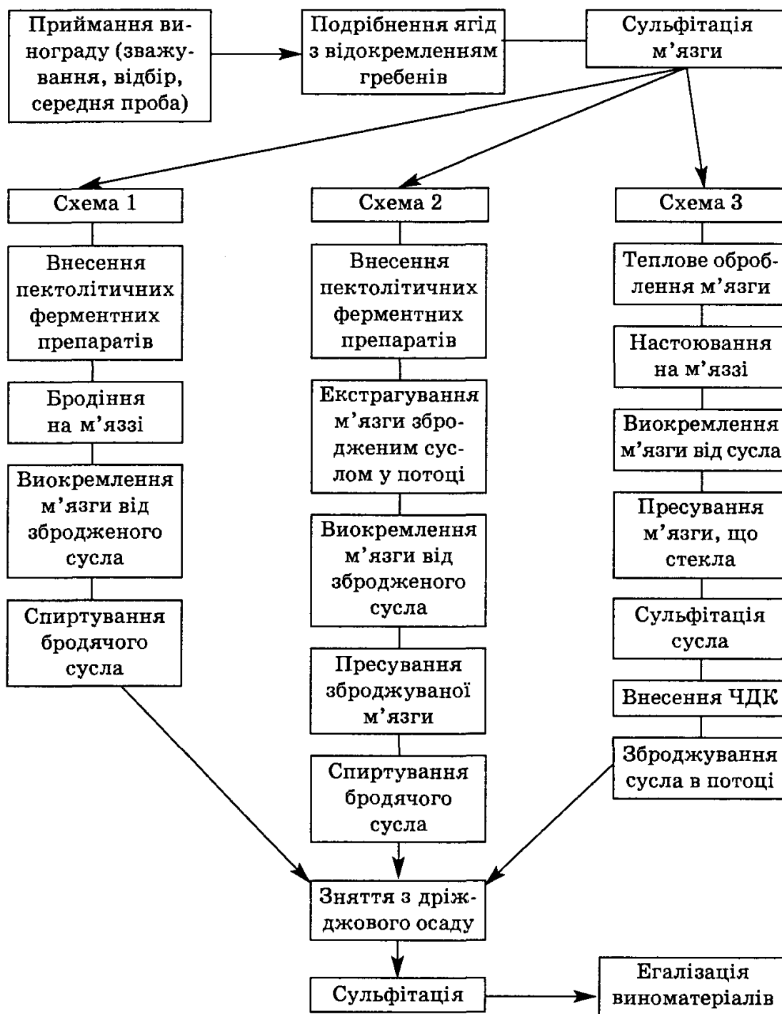
Рис. 22. — Технологічні стадії отримання виноматеріалів для білих і червоних вин спеціального типу
