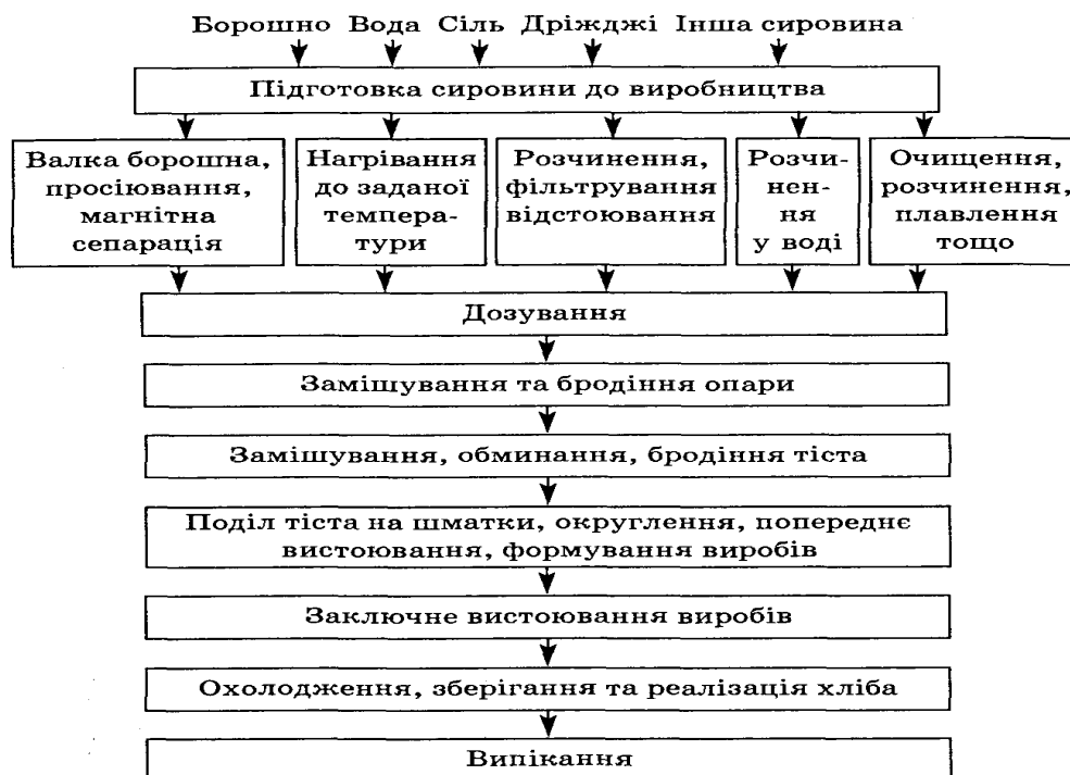
Рис. 3. — Принципово-технологічна схема виробництва хліба
