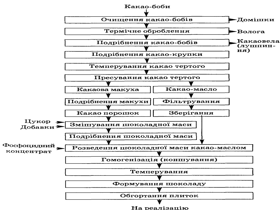
Рис. 11 — Технологічна схема виробництва шоколаду
