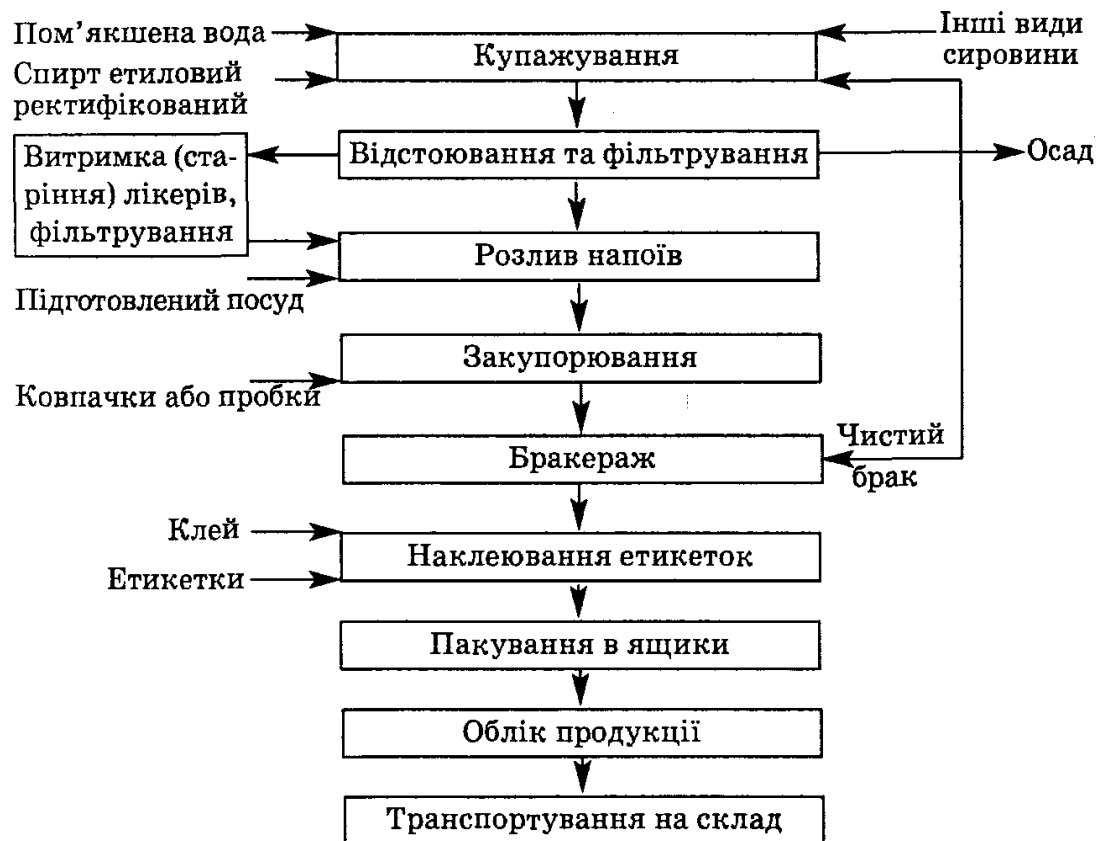
Рис. 19. — Принципово-технологічна схема виробництва лікєро-горілчаних напоїв
