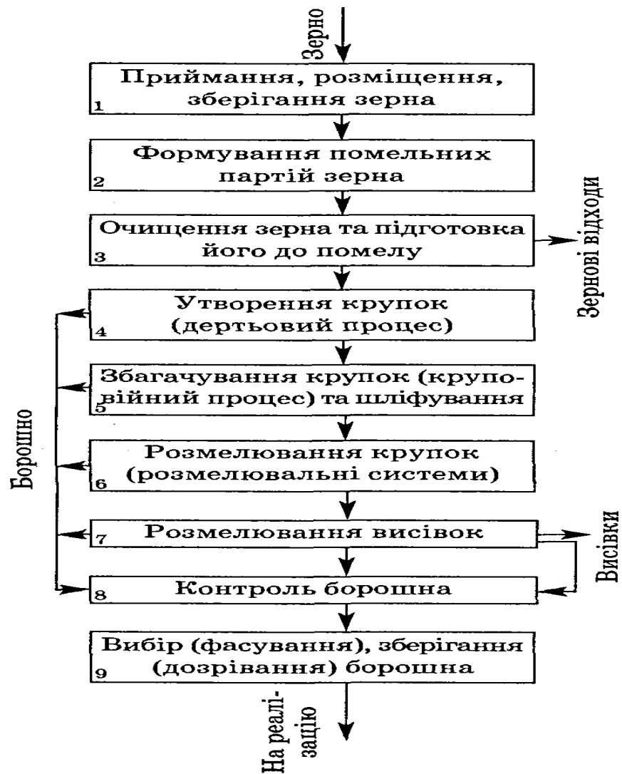
Рис. 1. — Принципово-технологічна схема виробництва борошна
