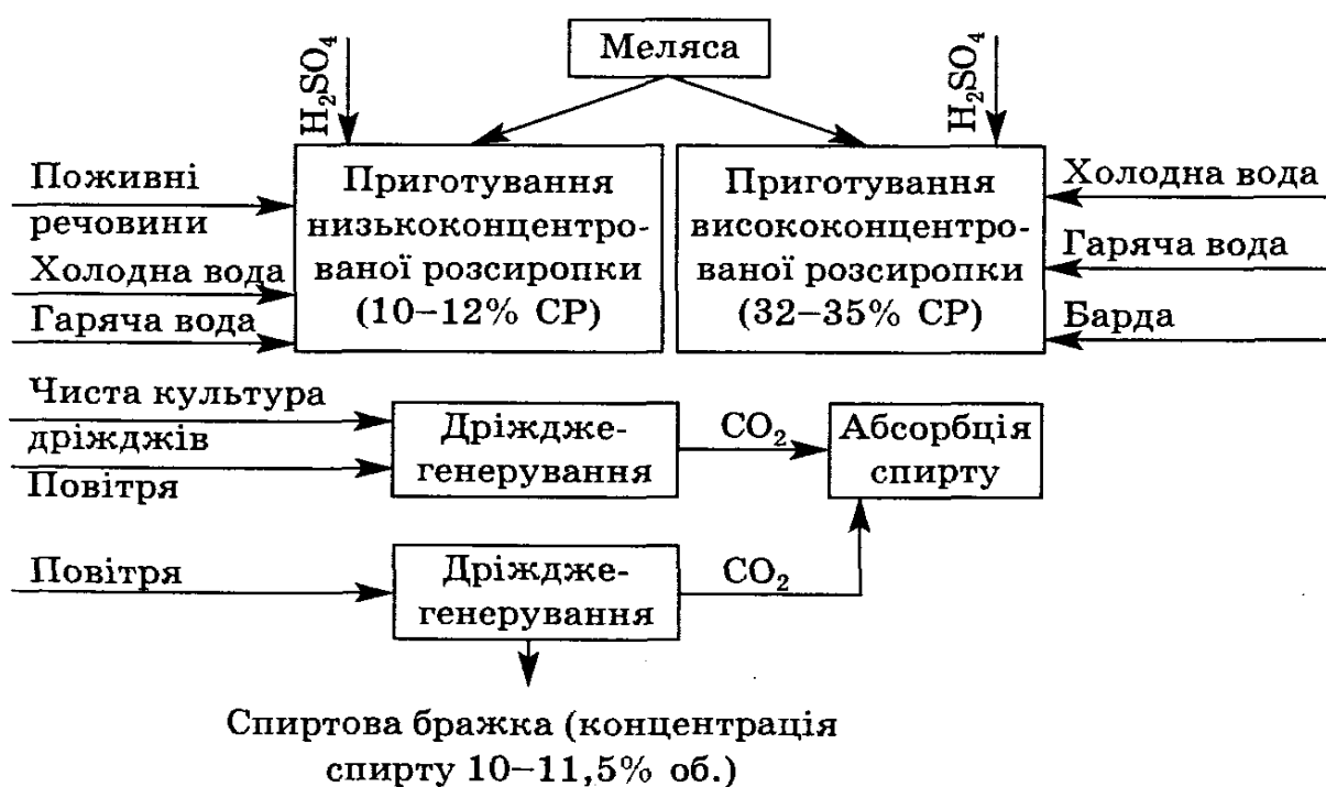
Рис. 17. — Принципова технологічна схема виробництва спиртової бражки з меляси
