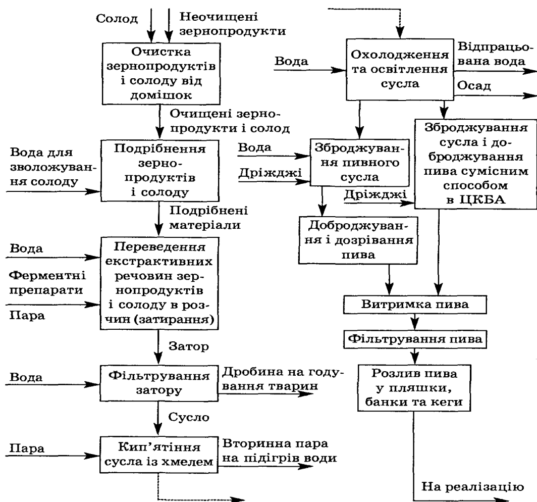
Рис. 27. — Принципово-технологічна схема виробництва пива
