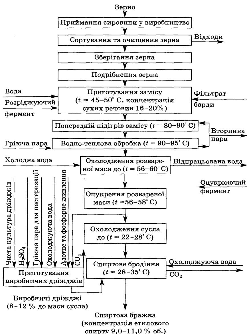
Рис. 16 — Технологічна схема приготування спиртової бражки із крохмалевмісної сировини
