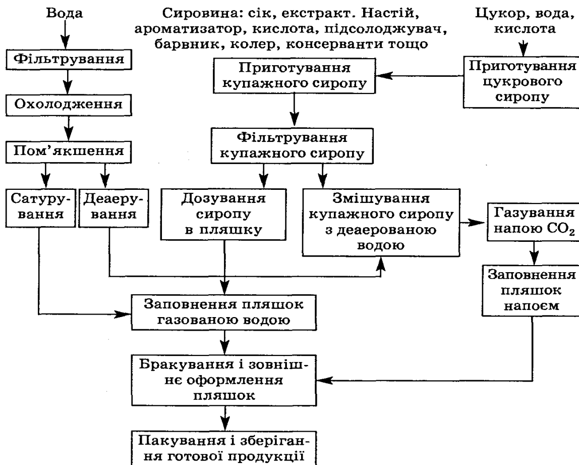
Рис. 28. — Принципово-технологічна схема виробництва безалкогольних напоїв
