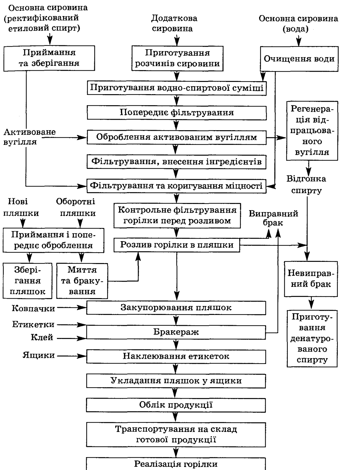
Рис. 18. — Принципово-технологічна схема виробництва горілки
