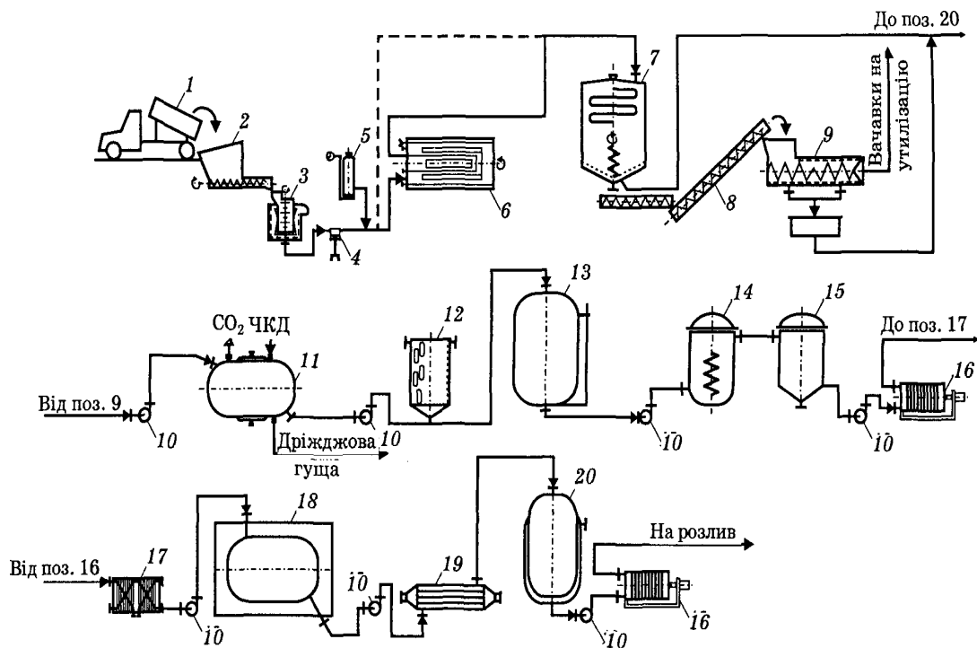
Рис. 25. — Апаратурно-технологічна схема виготовлення ординарнихміцних і десертних вин:
