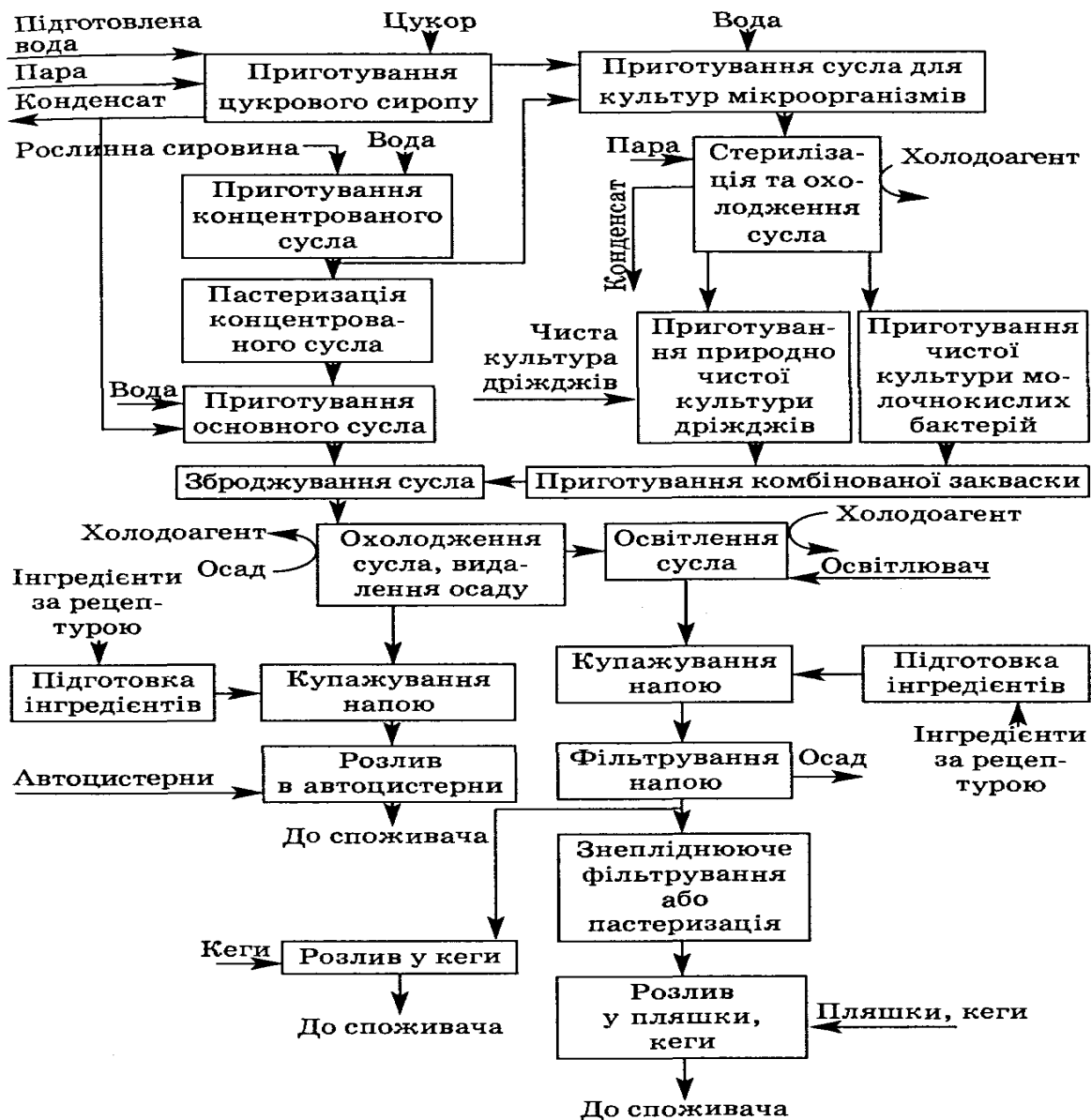
Рис. 29. — Технологічна схема виробництва ферментованих напоїв з використанням чистих культур дріжджів і молочнокислих бактерій і характерним ароматом житнього хлібу.
