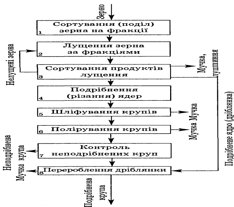
Рис. 2. — Технологічна схема лушильного відділення крупозаводу
