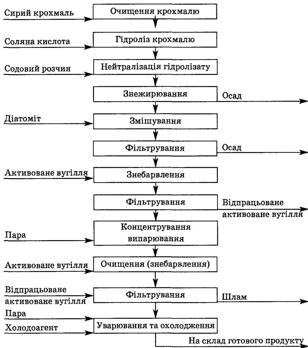
Рисунок 7. - Технологічн схема виробництва крохмальної патоки
