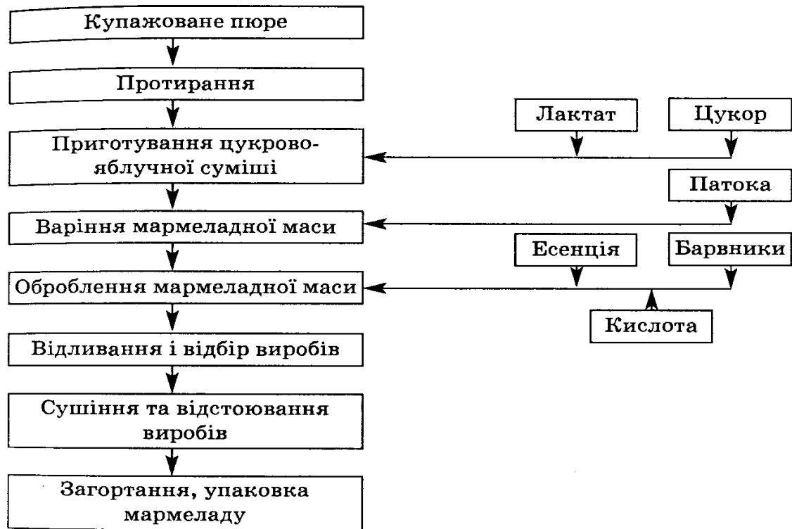
Рис. 14 — Технологічна схема виробництва яблучного мармеладу
