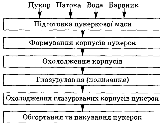
Рис. 13 – Функціональна схема виготовлення цукерок
