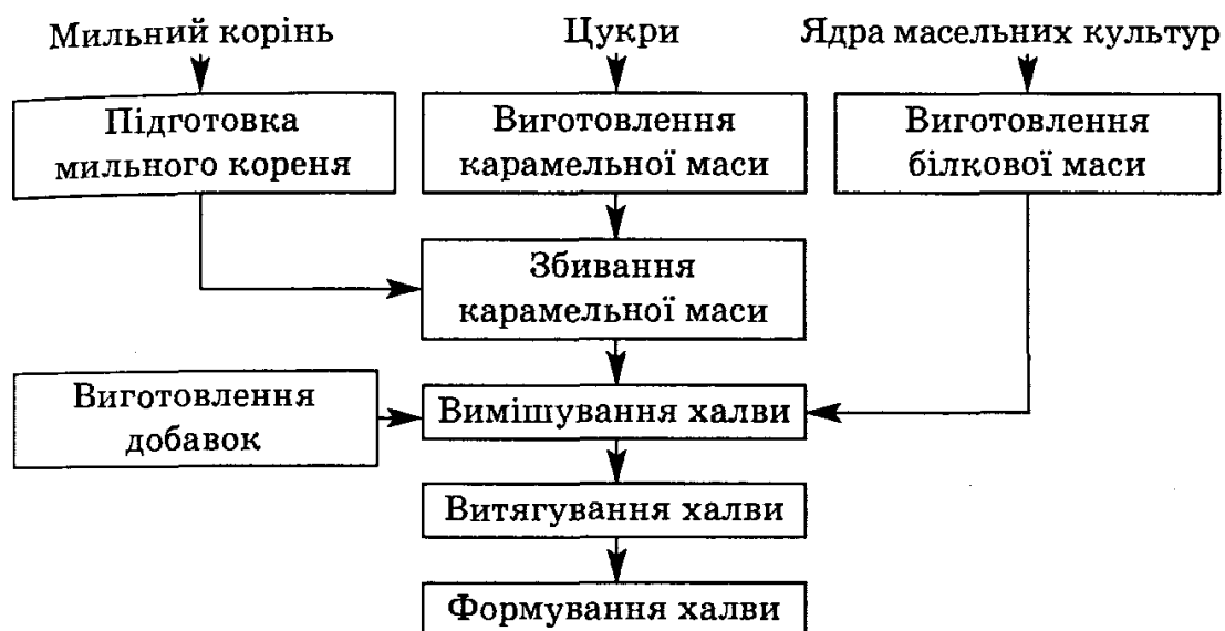
Рис. 15 — Принципово-технологічна схема виготовлення халви
