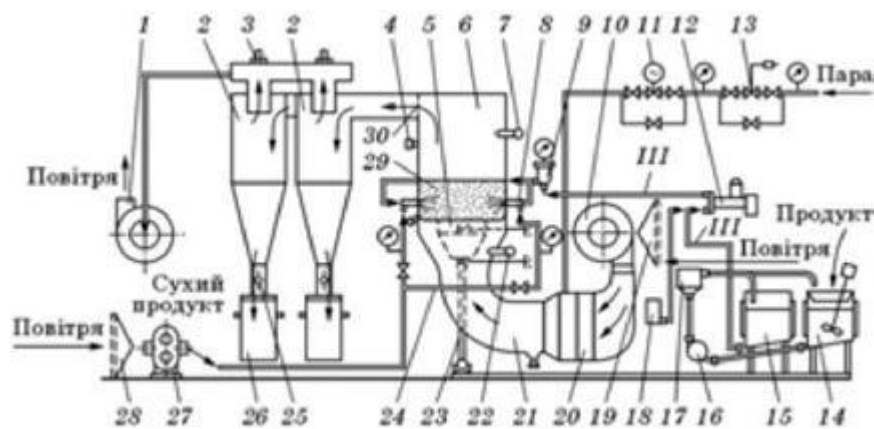
Рис. 30. - Схема сушарки А1-ФМУ:
