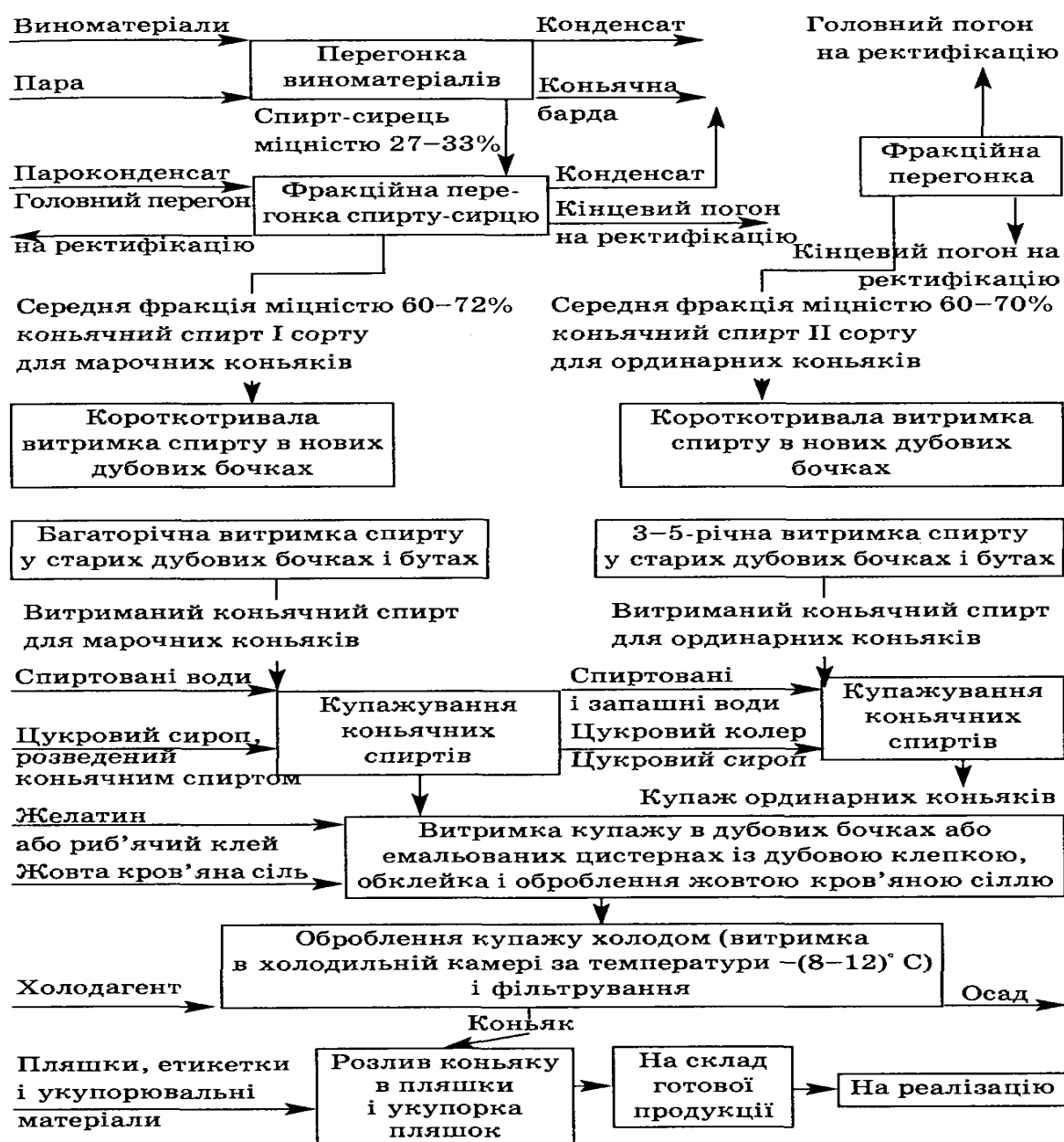
Рис. 26 — Технологічна схема коньячного виробництва
