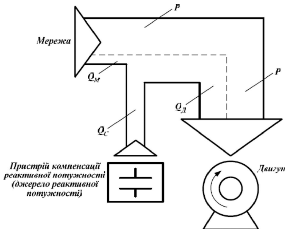
Рис.1.1 – Діагр.ама компенсації реакти.вної потужності: P - активна потужність;
