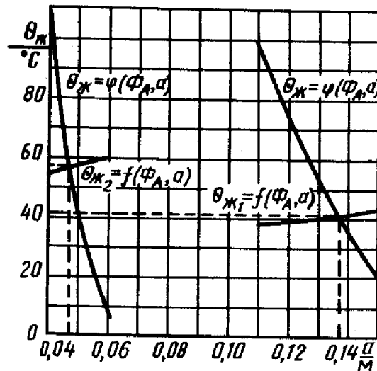
Рис. 9. Графічне вирішення рівнянь \theta_{ж}=f(\Phi_A, a) , \theta_{ж}=\varphi(\Phi_A, a) для нагрівального проводу при електрообігріві підлоги.
