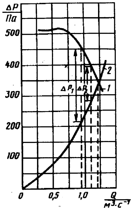
Рис.7. До визначення допустимого аеродинамічного опору роздаючих повітроводів:
