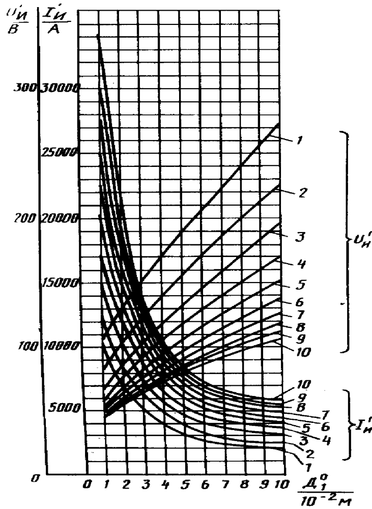
Рис.19. Залежність напруги U_i' на одновитковому індукторі і силі струму I_i' в індукторі від умовного діаметру D_1^0 індуктора (цифри у кривих вказують ширину індуктивного проводу в сантиметрах).
