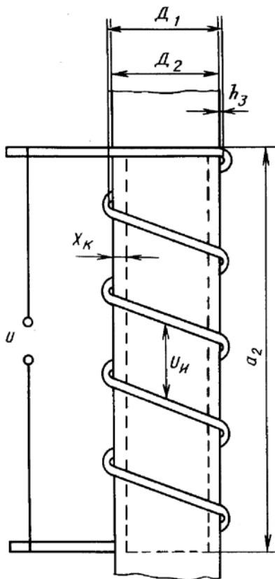
Рис.20. До розрахунку циліндричного індуктора
