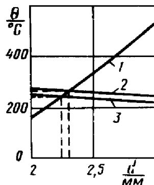
Рис. 14. Графічне вирішення рівнянь \theta=f(d) , \theta=\varphi(d) для сталюго дроту при електрообігріві парників: 1 - \theta_{не}=\varphi(d) ; 2 - \theta_{не \text{ ґрунту}}=\varphi_2(d) ; \theta_{не \pi}=\varphi_1(d) .
