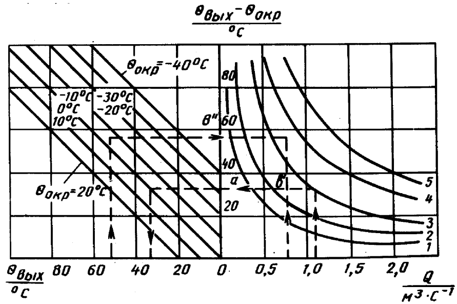
Рис.6. Номограма для визначення температури повітря, яке виходить з еоелектрокалориферних установок СФОЦ:
