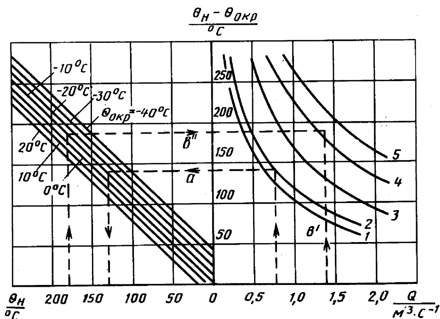
Рис.5. Номограма для визначення температури ТЕНа в електрокалориферних установках серії СФОЦ:
