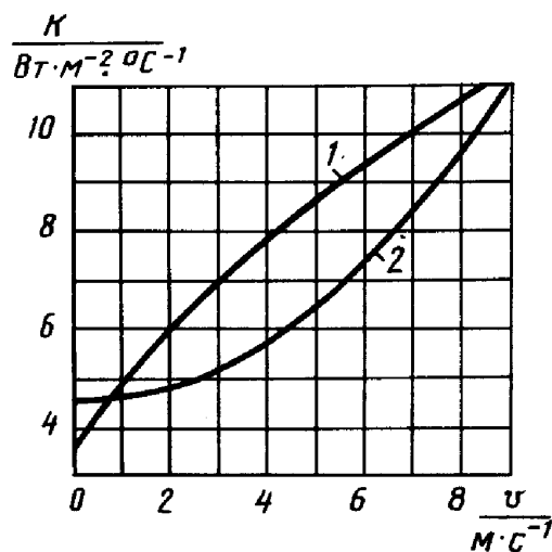
Рис.10. Значення приведенного коефіцієнта теплопередачі через скління теплиць (1) і парників (2) при різній швидкості вітру.
