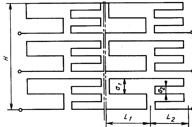
Рис. 8. До розрахунку електронагрівної підлоги в свинарнику-маточнику.
