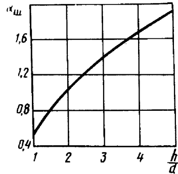
Рис. 1. Залежність коефіцієнту \alpha_w від відношення h/d для дротового спірального електронагрівача.
