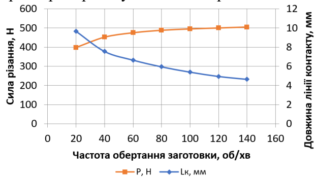
Рисунок 3 – Залежності колової складової сили різання і лінії контакту шліфувального круга від частоти обертання заготовки
